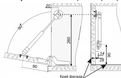
Схема установки газлифта секретерного
