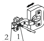
Регулировка створки по ширине
