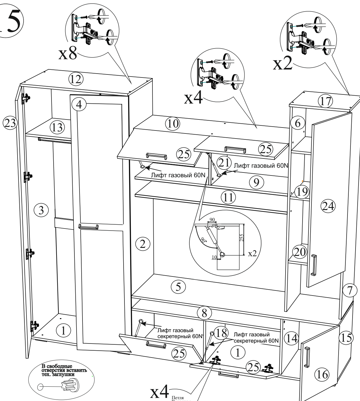
Схема установки газлифта секретерного
