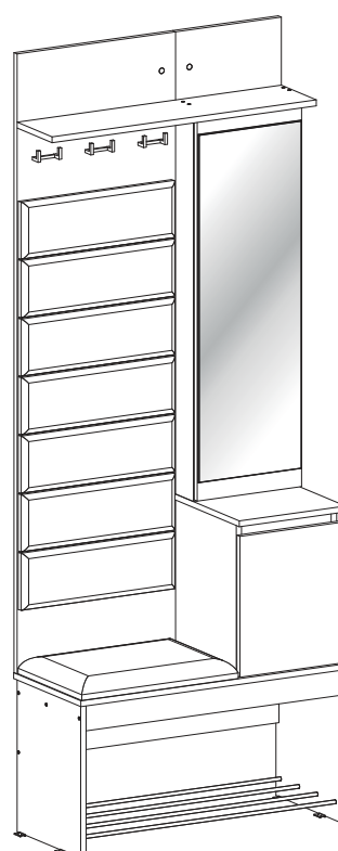
Правосторонняя сборка
