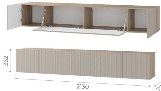
Навесной шкаф ШКН-03 (max нагрузка на верхнюю крышку - 10 кг, max нагрузка на полку - 10 кг)
