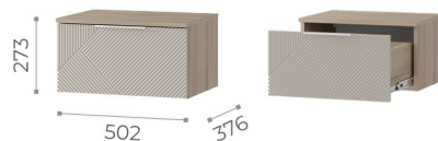
Тумба прикроватная ТБ-11 (max нагрузка на ящик - 5 кг)
