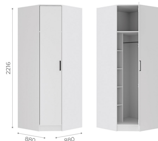
Шкаф угловой ШКУ-04 (max нагрузка на полку / штангу - 10 кг)
