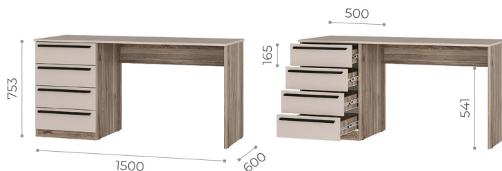
Стол письменный ПС-05
