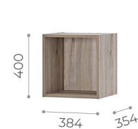
Полка навесная АН-05
