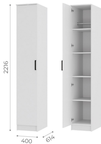
Пенал ПН-07 (max нагрузка на полку / штангу - 10 кг)
