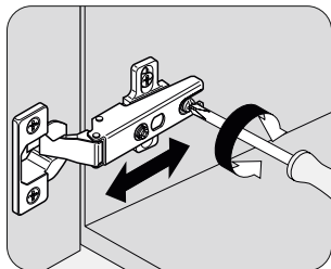
Схема регулировки петель
