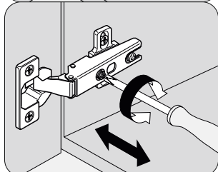
Схема регулировки петель
