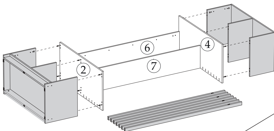
Левосторонняя сборка
