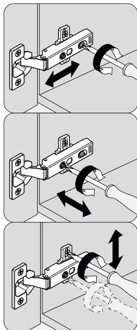
Схема регулировки петель Z
