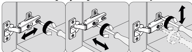
Схема регулировки петель J
