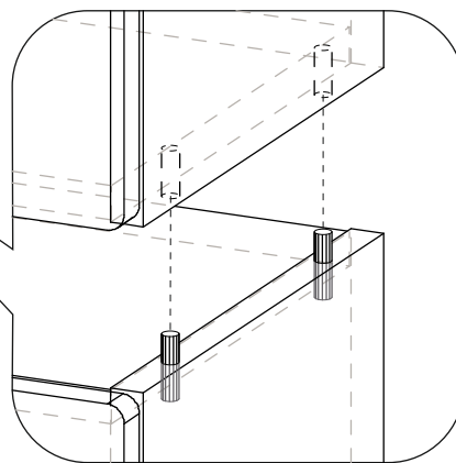
Шкаф навесной "Пандора" ШКН-16
