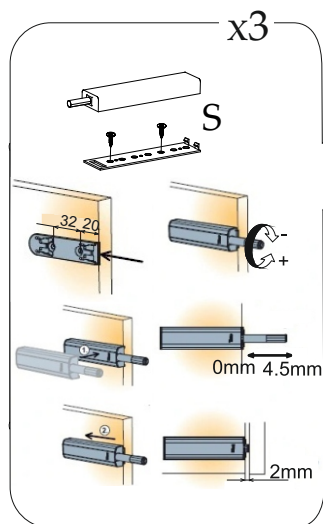
Схема крепления толкателя фасадов
