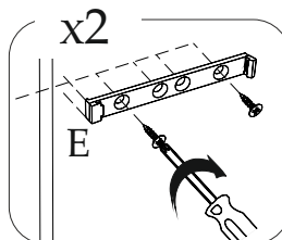
Схема крепления толкателя фасадов
