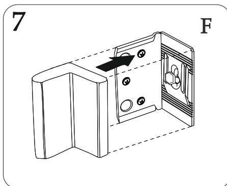
Регулировка толкателя
