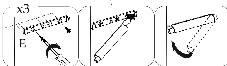
Схема крепления толкателя фасадов
