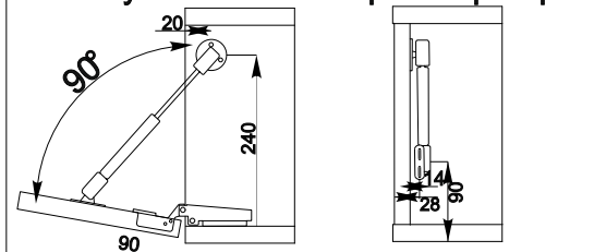
Схема установки газлифта секретерного
