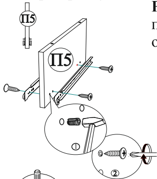
Рис.2 Прикручивание направляющих на перегородку П5
