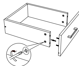
Рис.11 Установка выдвижных ящиков
