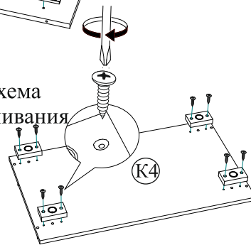
Рис.4 Схема расстановки шкантов и эксцентриковых стяжек
