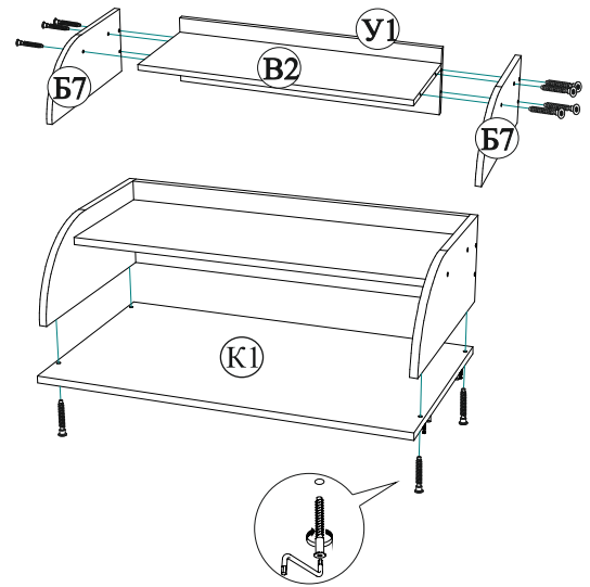
Рис.6 Сборка корпуса комода
