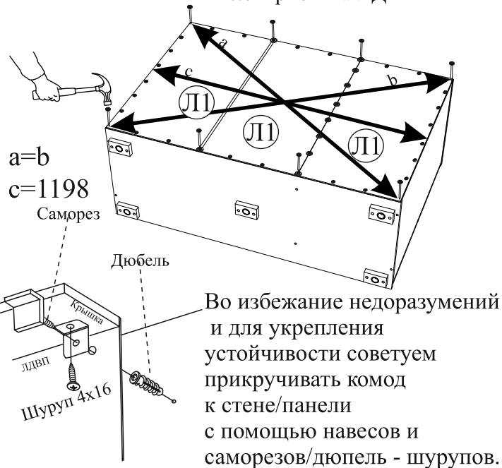
Рис.7 Прибивка ЛДВП
