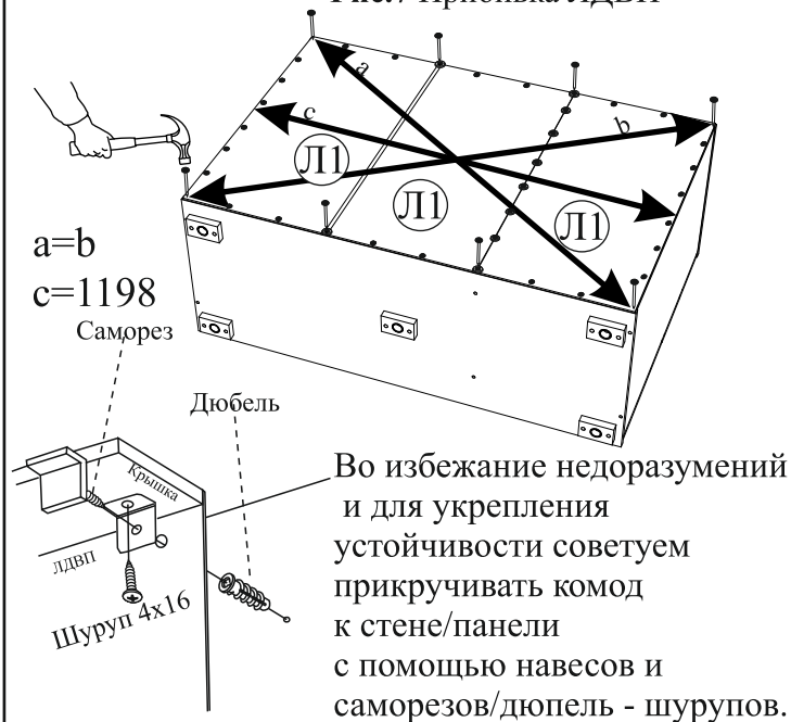
Рис.7 Прибивка ЛДВП
