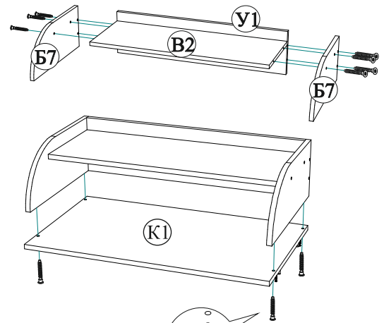
Рис.5 Сборка надстройки комода
