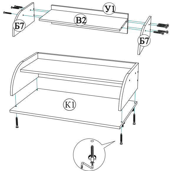
Рис.5 Сборка надстройки комода
