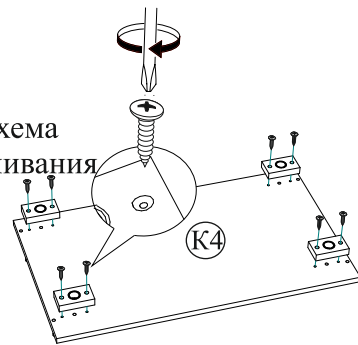
Рис.4 Схема расстановки шкантов и эксцентриковых стяжек
