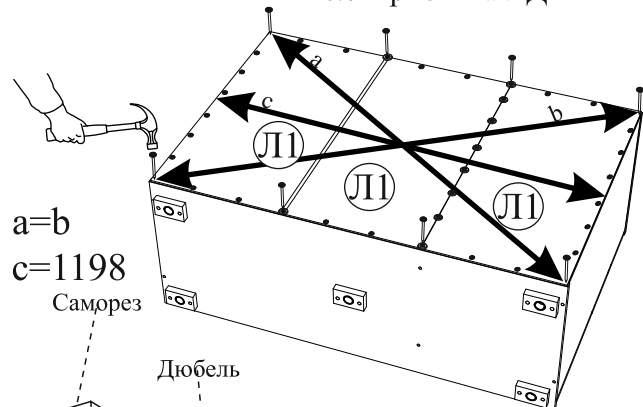
Рис.7 Прибивка ЛДВП
