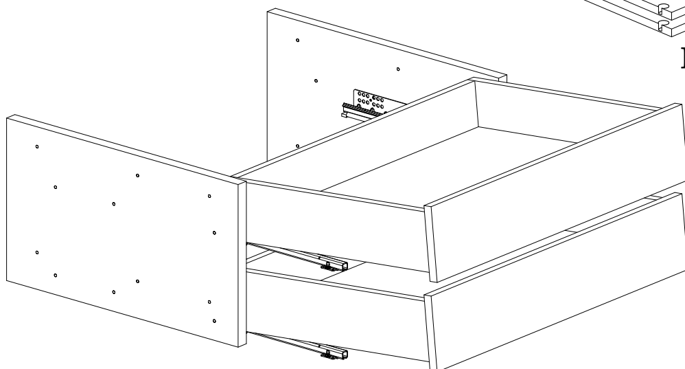
Ящики СМ "Тринити" ШК-21
