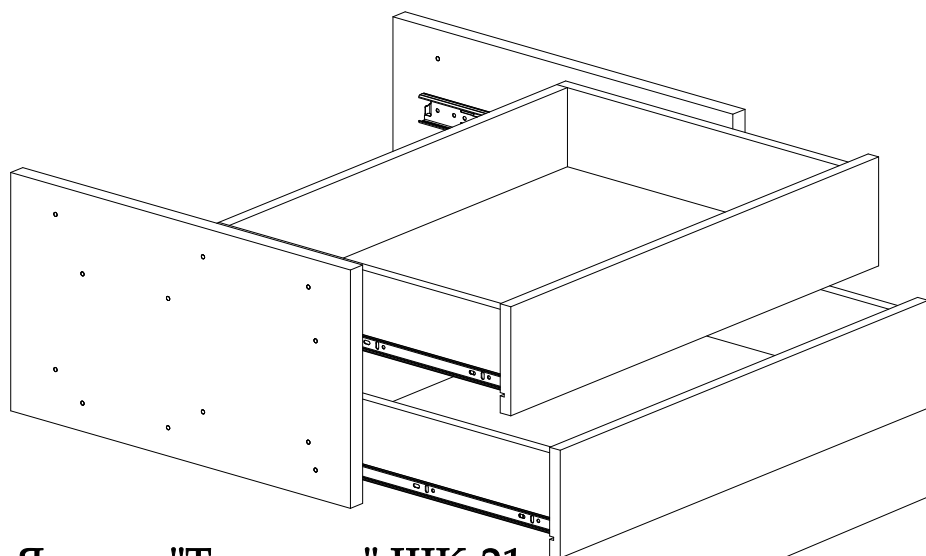
Ящики "Тринити" ШК-21
