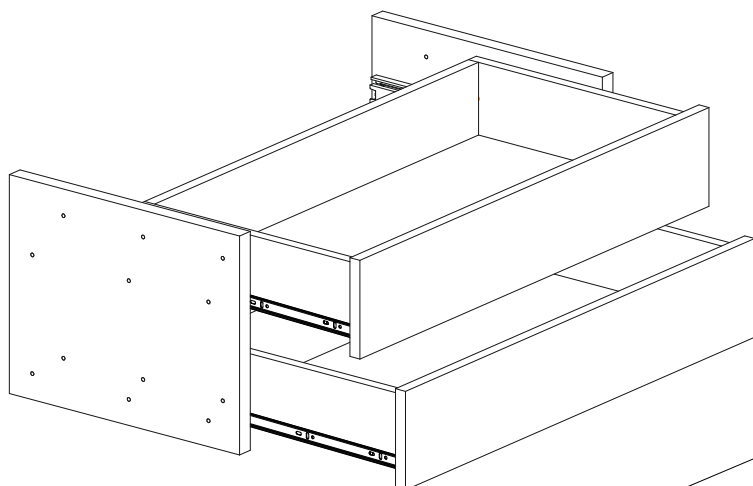
Ящики "Тринити" ШК-22 Лайт
