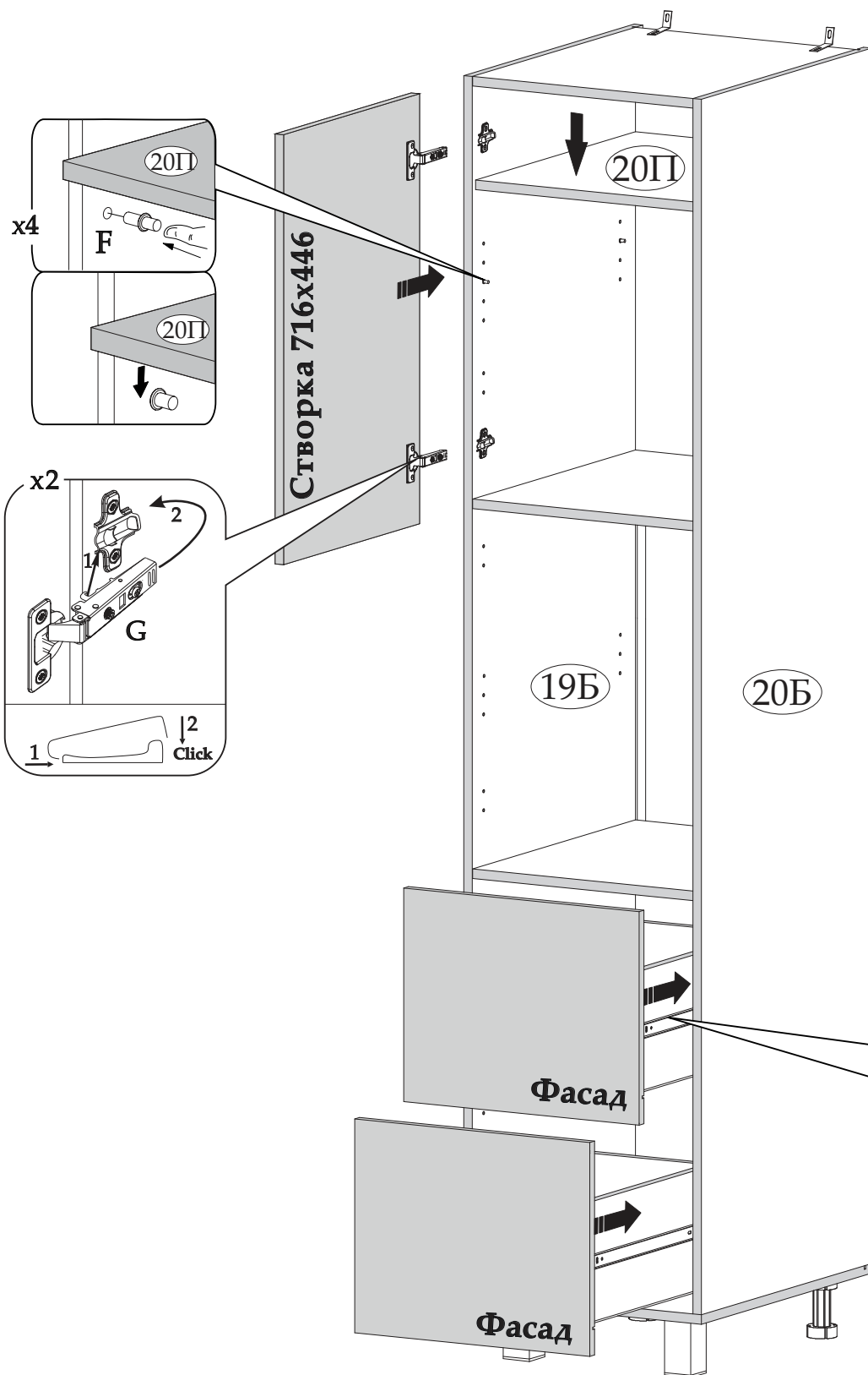
Схема регулировки петель
