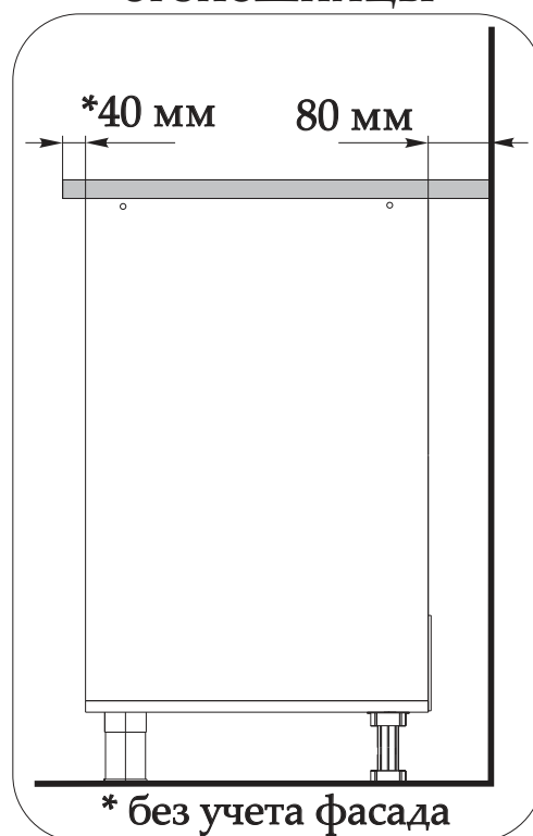
Схема установки столешницы
