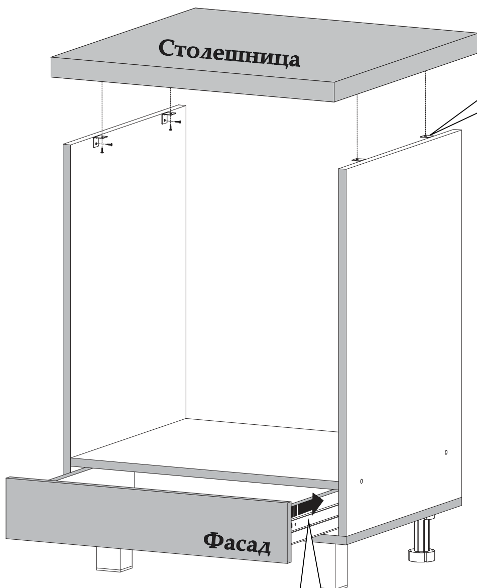
Схема установки столешницы
