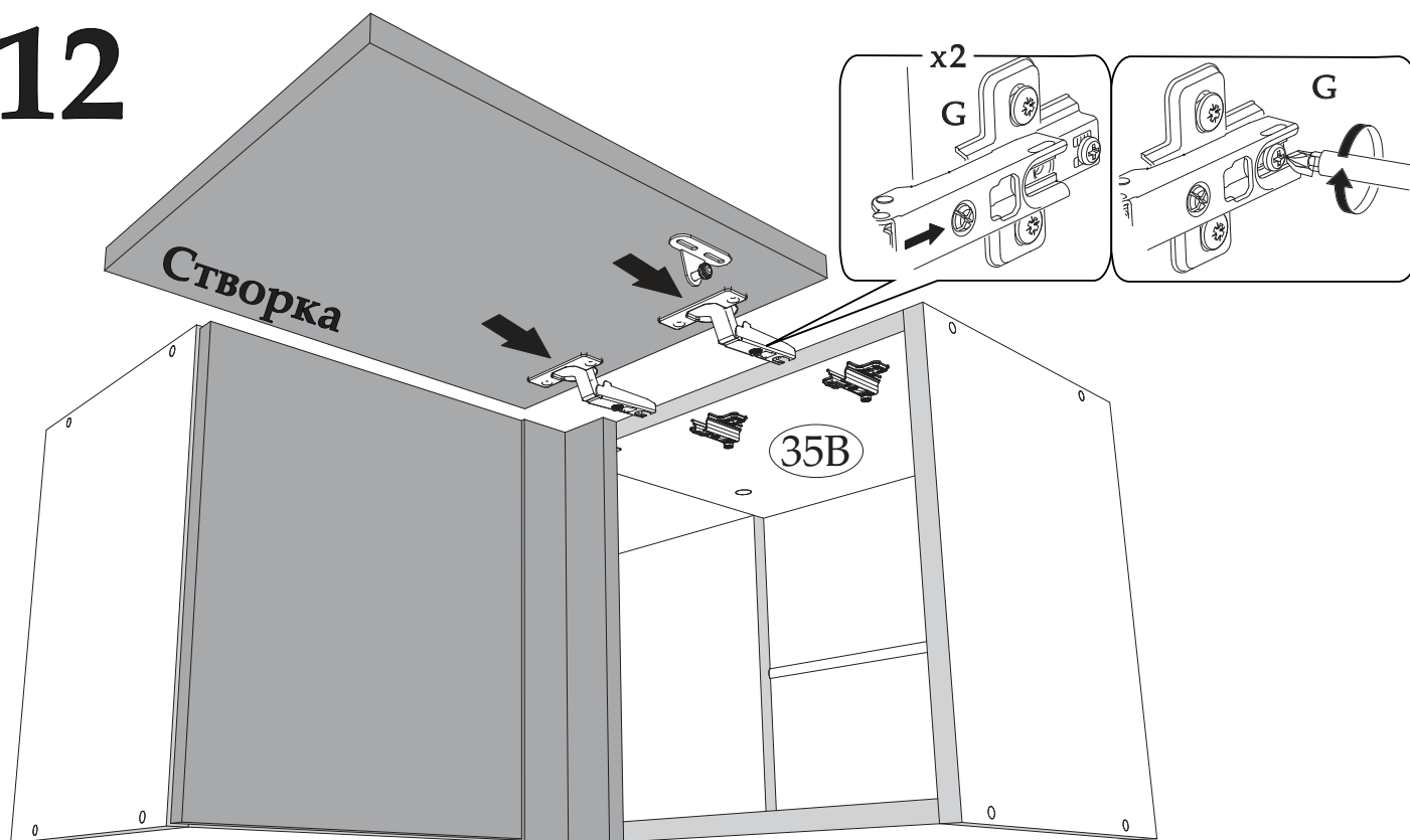
Схема регулировки петель
