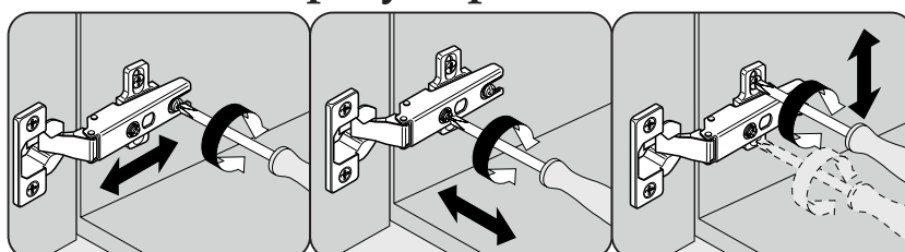
Схема регулировки петель
