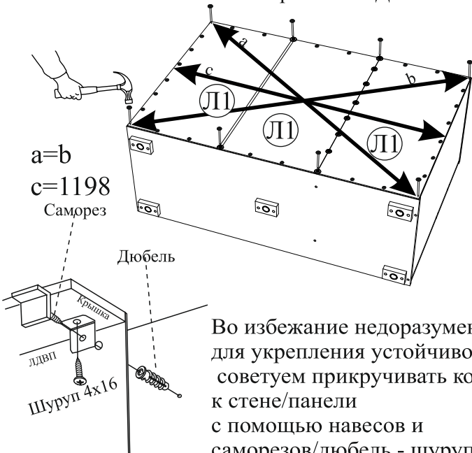
Рис.7 Прибивка ЛДВП
