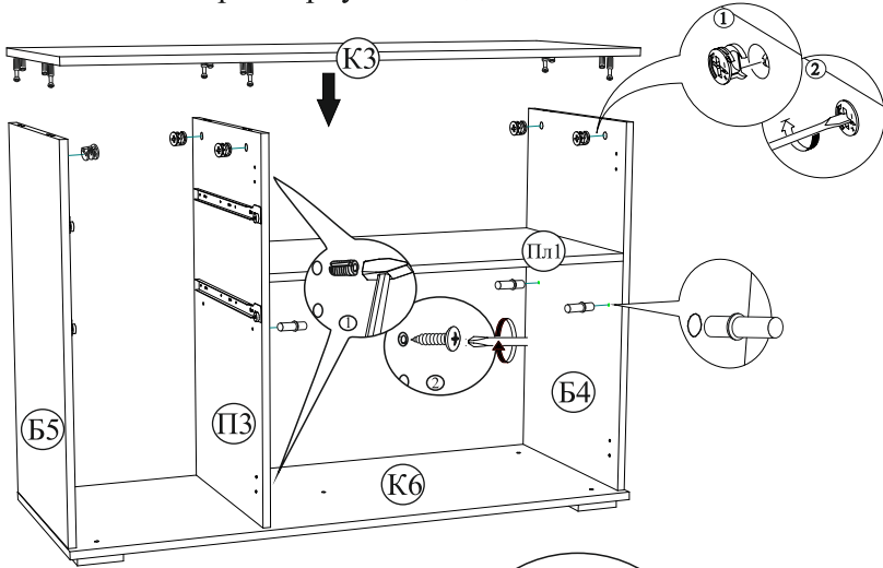
Рис.6 Регулировка опор
